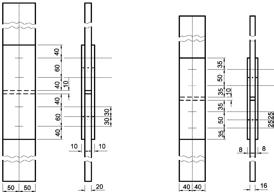
а) болти M20 в отворах діаметром 22 мм M20 bolts in 22 mm diameter holes
