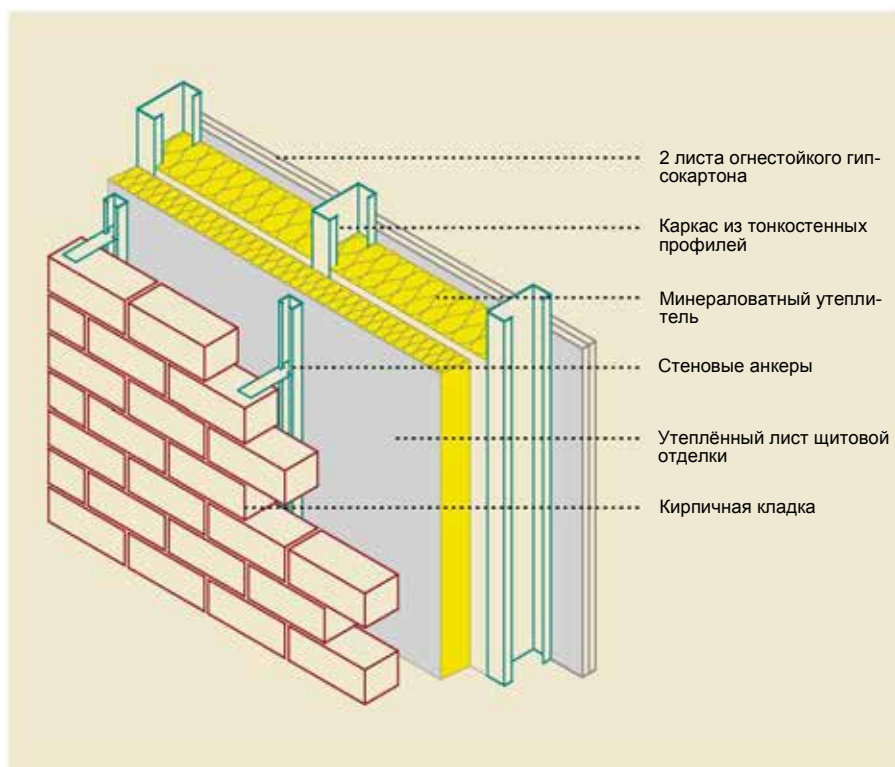
Рисунок 7.3 Внешняя стена с кирпичной кладкой, прикрепленной к каркасу из тонкостенных стальных профилей
