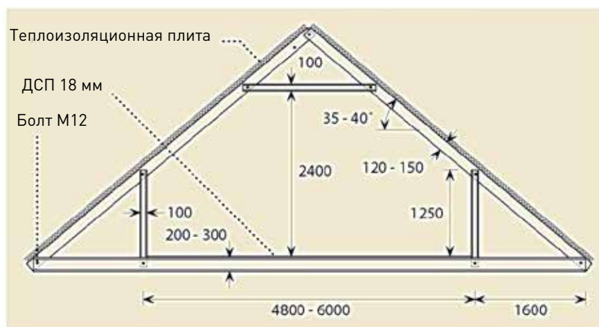
Рисунок 7.7 Система «открытой крыши» с каркасом из тонкостенных стальных профилей
