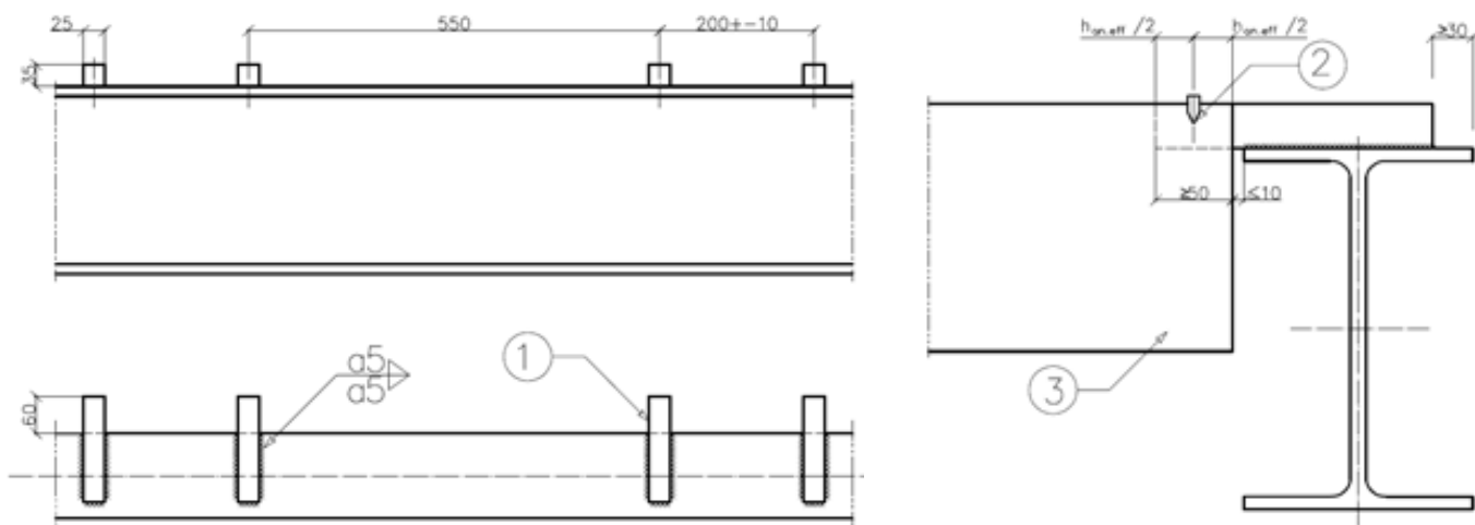
Рис. 5.4. Приклад вузла приєднання насталу до опорного столика за допомогою дюбель-піроцвяхів: 1 – сталевий опорний столик із суцільного квадратного перерізу С235, 2 – дюбель-піроцвях для кріплення насталу до столика, 3 – профіль TRP-200
