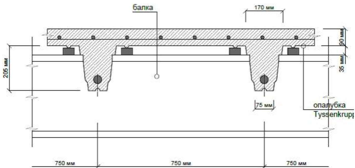
Рис. 5.3. Визначення розрахункового прольоту насталу L і деталь типового кріплення до опорного столика
