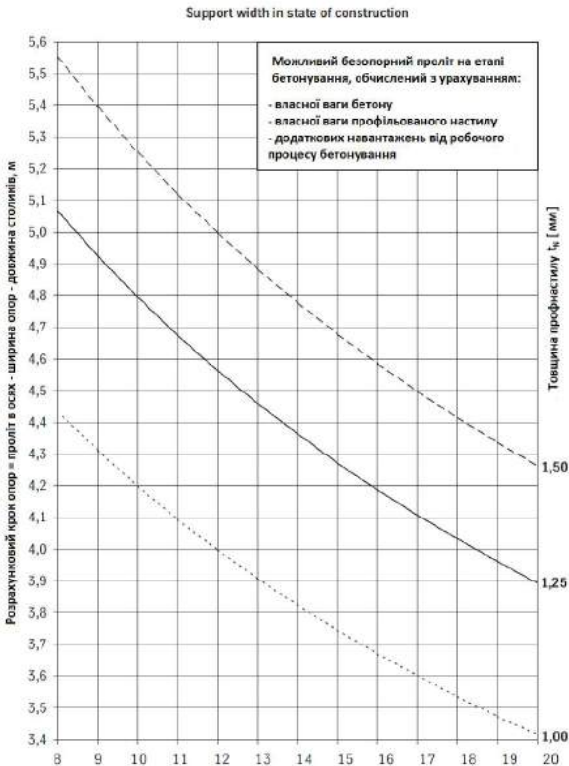
Рис. 5.5. Визначення товщини профлиста типу TRP-200 при використанні у якості безопорної опалубки в перекритті при різних прольотах на етапі зведення
