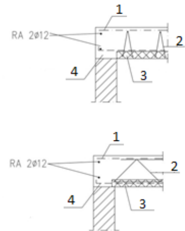
Рис. 3.3. Рішення з філігранними плитами як опалубкою для монолітних плит по сталевих балках: 1 – верхня арматура, 2 – просторові каркаси, 3 – філігранна плита, 4 – анкетування поздовжнього армування
