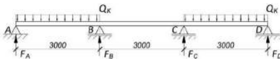
Рис. 5.30. Розрахункова схема плити для обчислення прогину при дії корисного навантаження в двох прольотах
