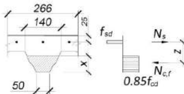
Рис. 5.27. Урахування верхнього армування у плиті (Рисунок 9.7 ДСТУ-Н Б EN 1994-1-1)
