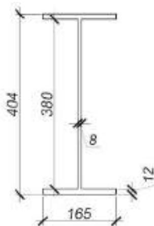
Рис. 5.34. Схема перерізу балки
