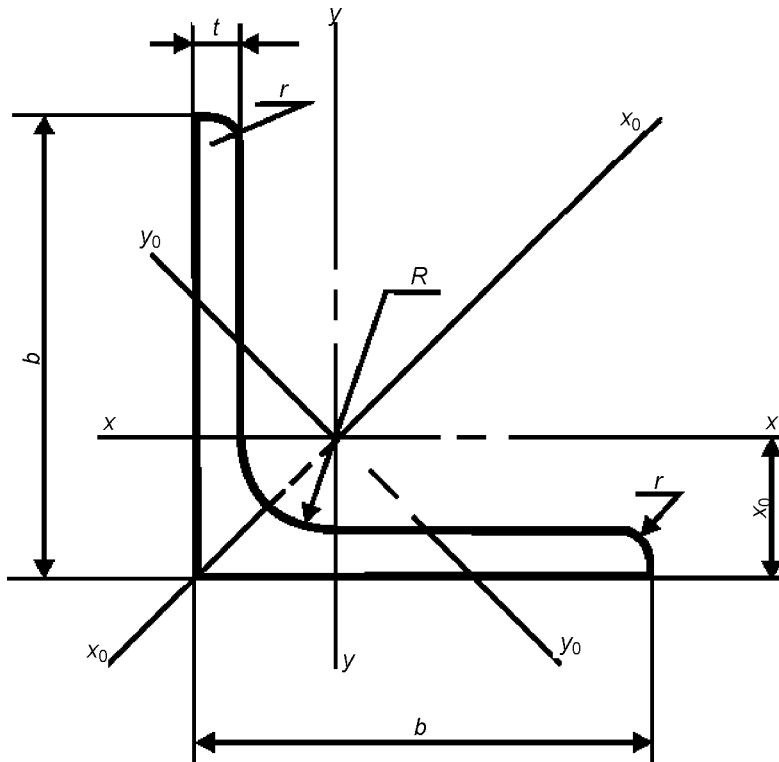
Рисунок 1 — Поперечний переріз рівнополічних кутиків
