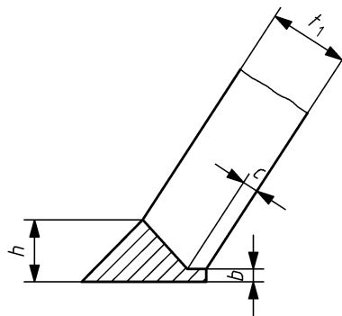
Деталь С:
