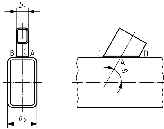
Деталь С:
