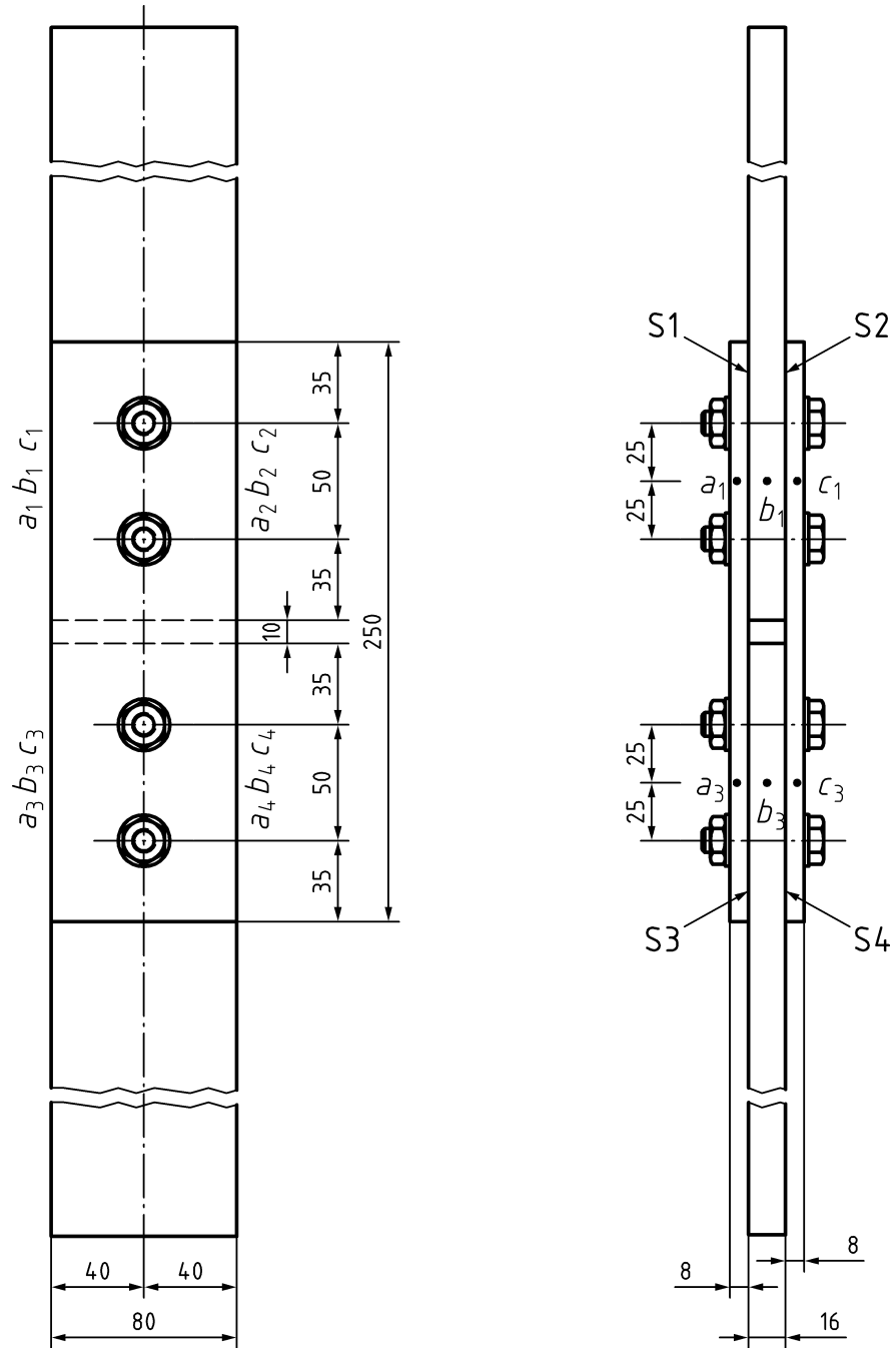
б) Болти М16, встановлені в отвори діаметром 18 мм
