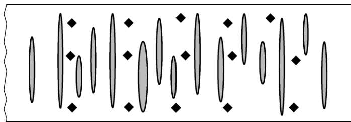
Рисунок D.4 – Місця вимірювання на відшліфованій поверхні газополуменевого різку
