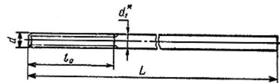
Поз. 7 ( d = 12 - 48 мм)
