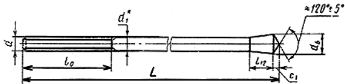
Поз. 10 ( d = 12 - 48 мм)
