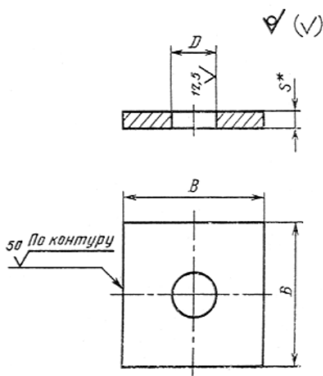
Плита анкерная (поз. 11 по черт. 1)
