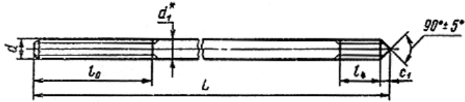
Поз. 9 ( d = 12 - 48 мм)
