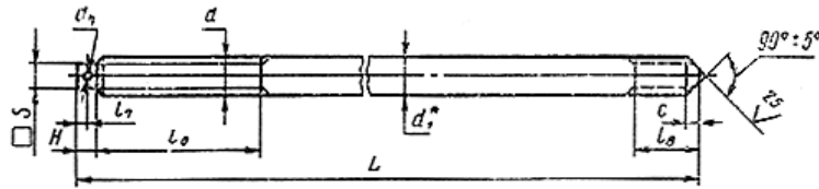
Поз. 5 ( d = 24 - 64 мм)
