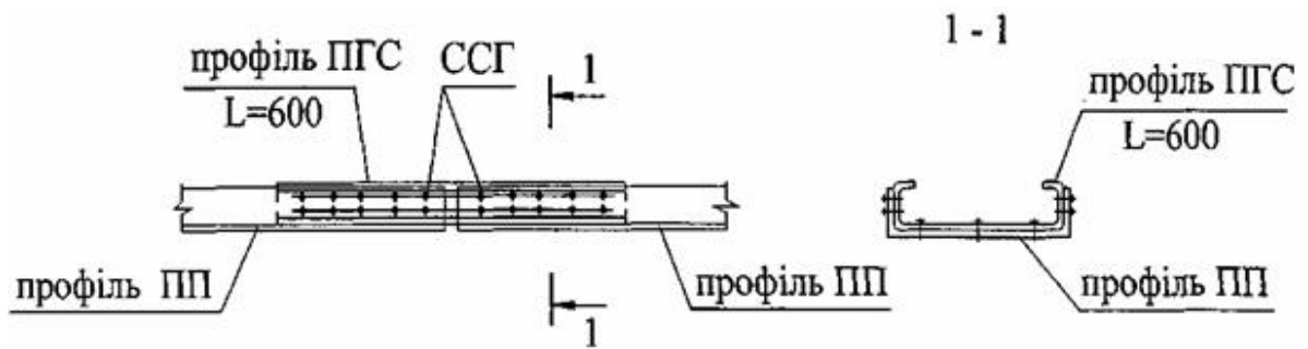
Рисунок 9.5 – Вузол 2
