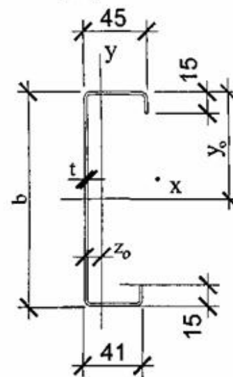
Профілі ПГС
