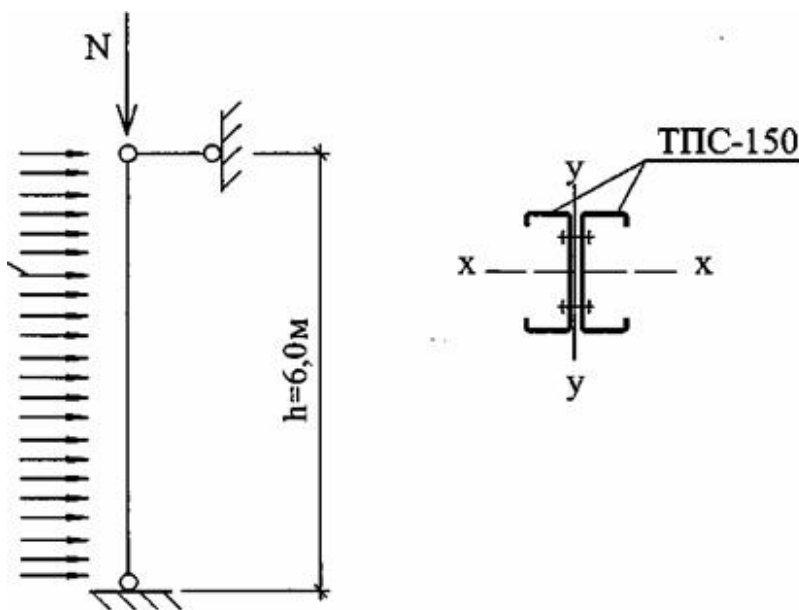
Рисунок В.7 – Розрахункова схема та переріз стояка стіни
