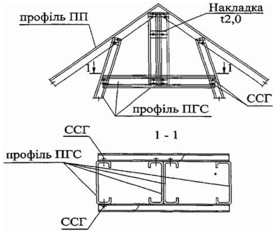
Рисунок 9.4 – Вузол 1
