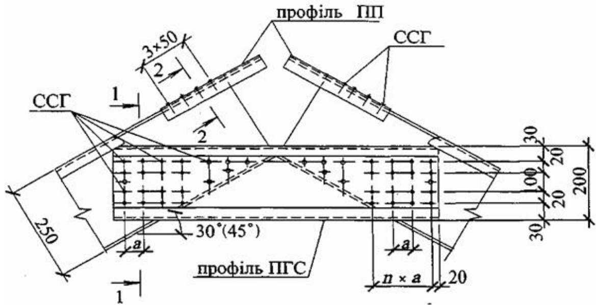
Рисунок 9.10 – Вузол 1
