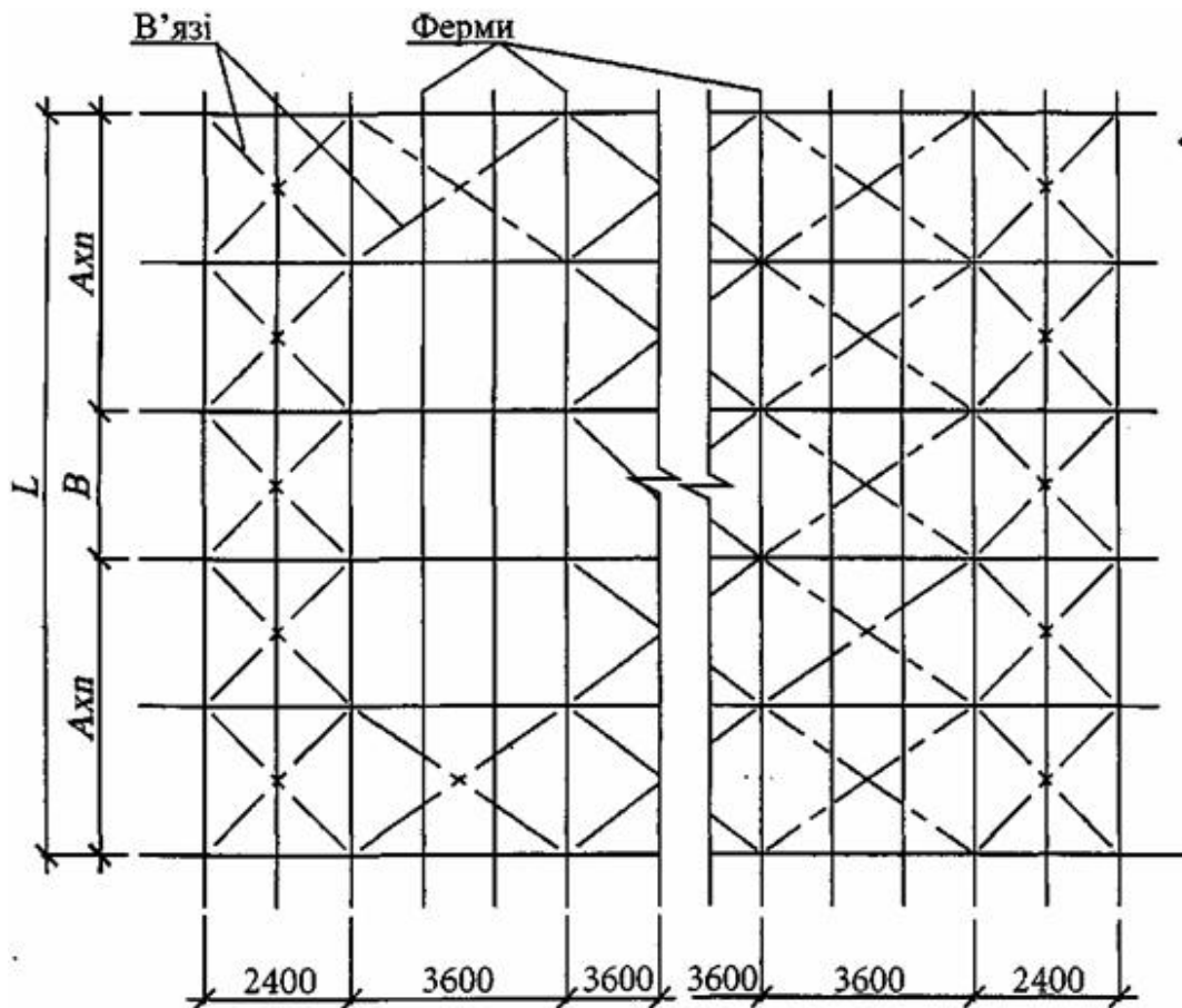
Рисунок 10.1 – Схема в'язей по нижніх поясах ферм
