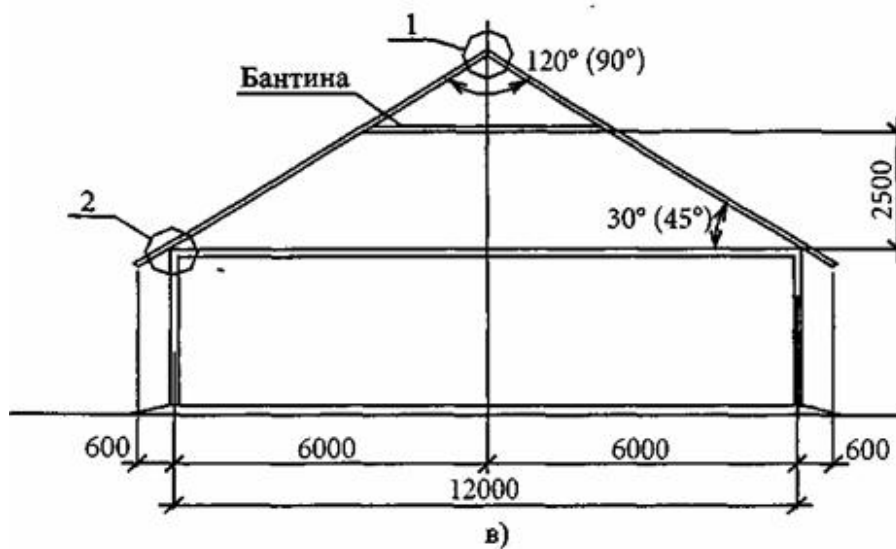
Рисунок 9.9 – Кроквяні балки
