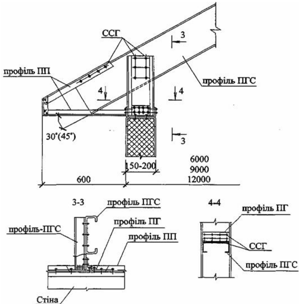
Рисунок 9.11 – Вузол 2
