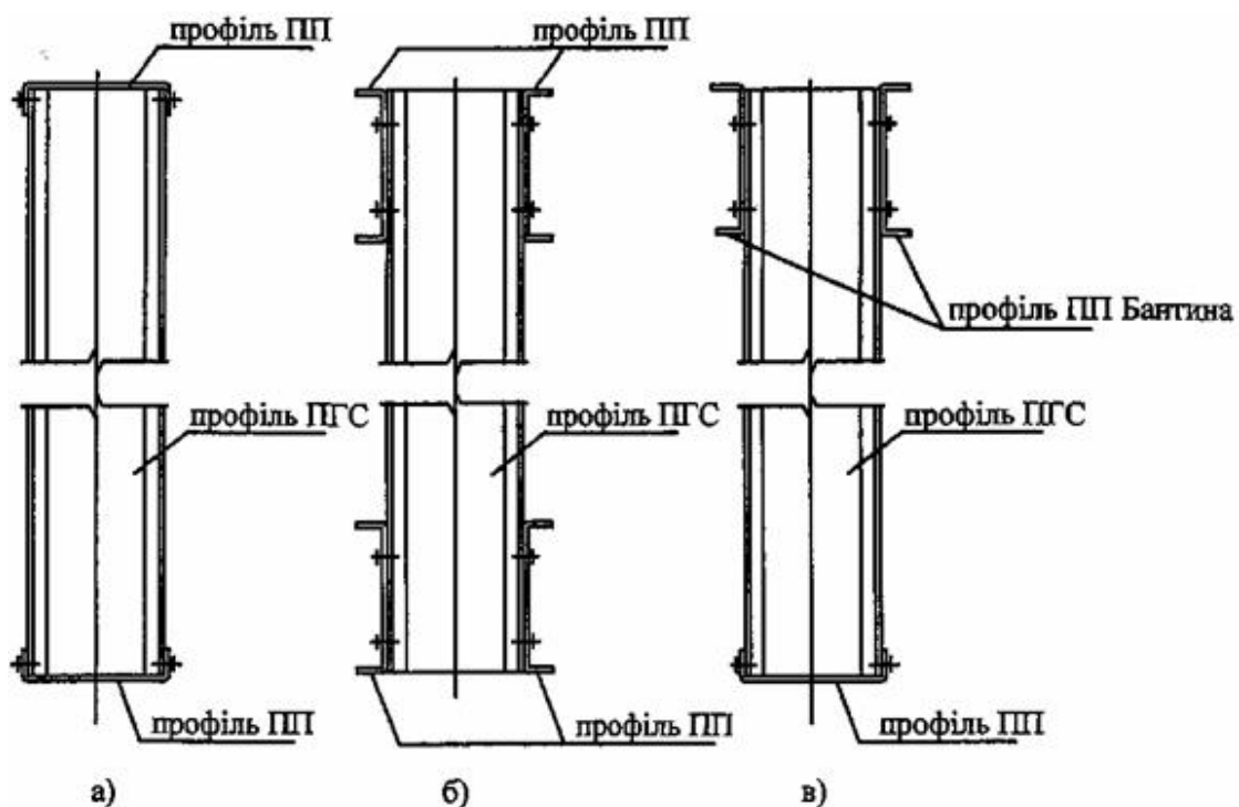
а, б, в – варіанти виконання верхнього та нижнього поясів ферм Рисунок 9.3 – Розріз 1-1
