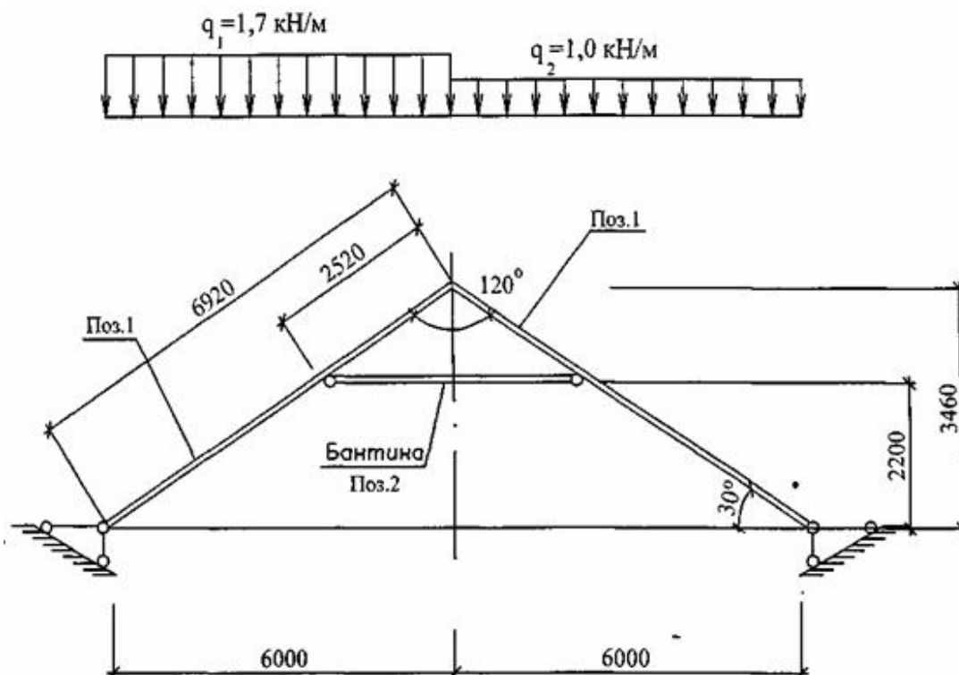
Рисунок В.6 – Розрахункова схема кроквяної системи
