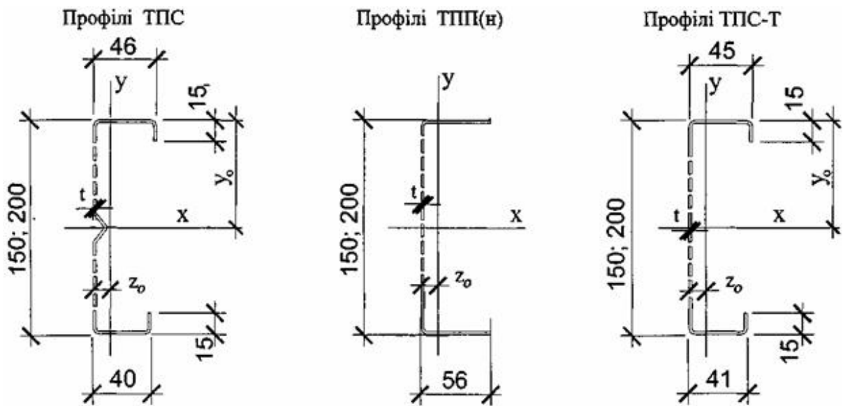
Рисунок А.1 – Перерізи профілів марок: ШП, ПП, ПС, ТПС, ТПП(н), ТПС-Т
