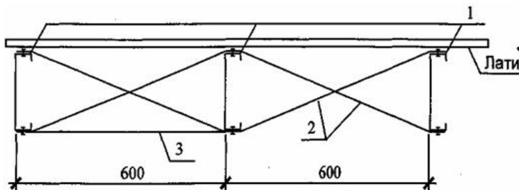
Рисунок 10.2 – Система хрестових в'язей для балок (прогонів)
