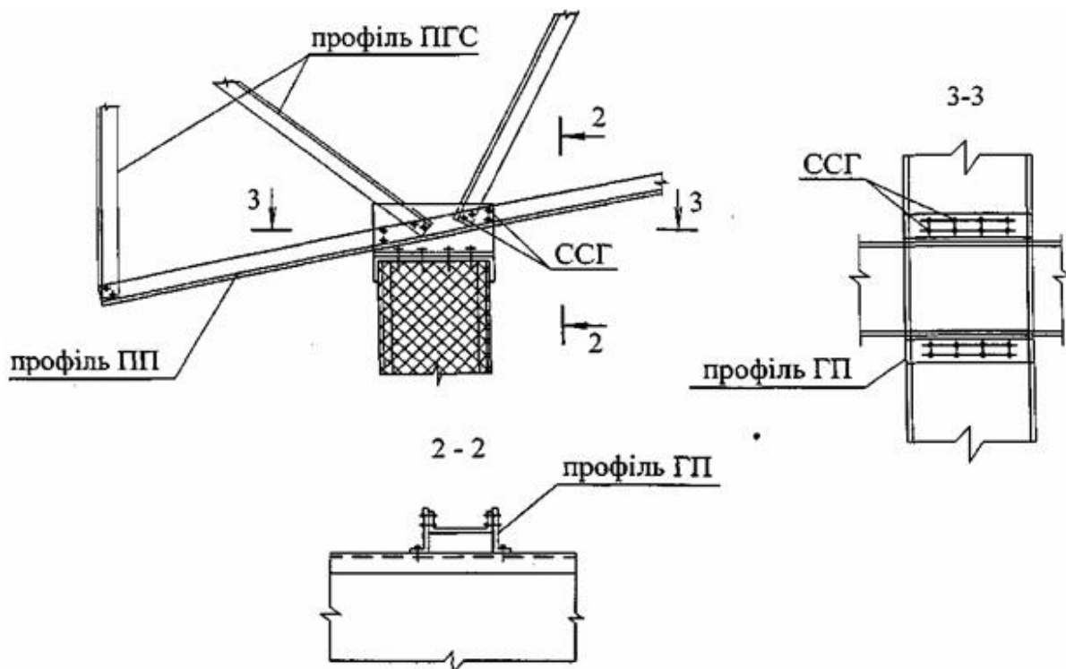
Рисунок 9.8 – Вузол 5
