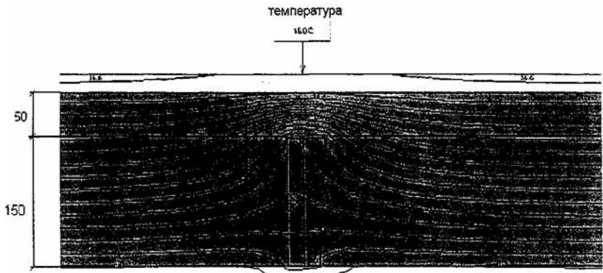
Рисунок 13.2 – Температурне поле зовнішньої стінової панелі з двохаровою теплоізоляцією завтовшки 150 + 50 мм (горизонтальний переріз)
