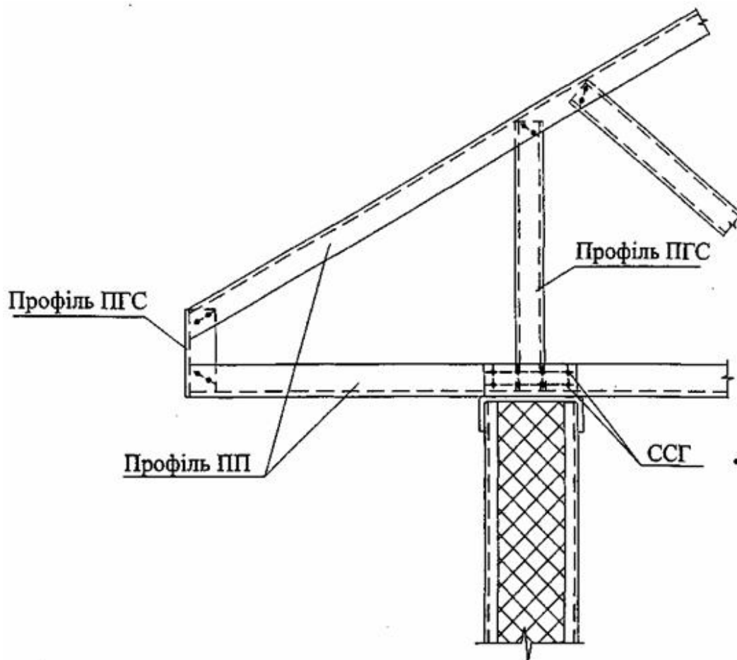
Рисунок 9.6 – Вузол 3
