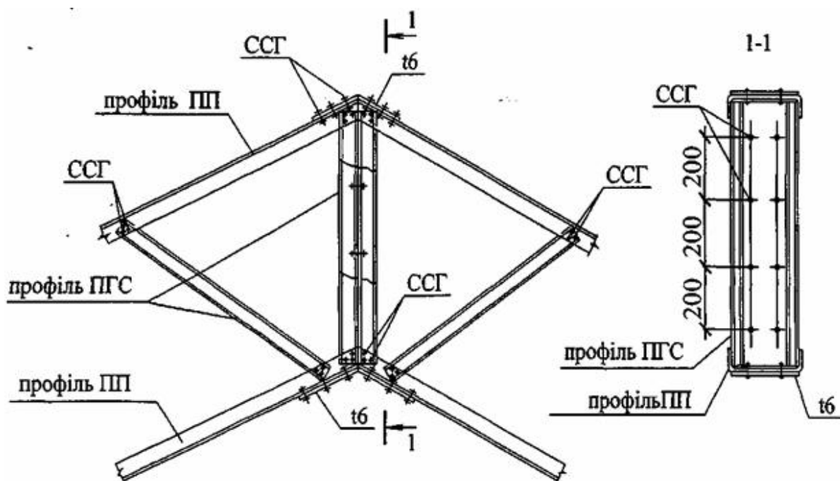
Рисунок 9.7 – Вузол 4
