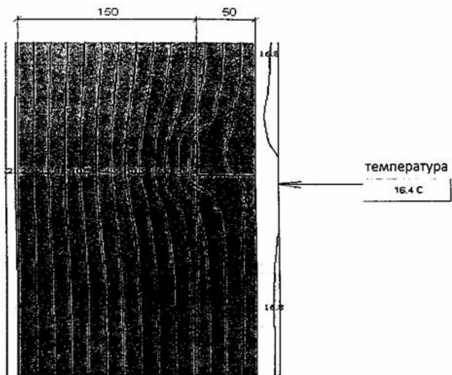
Рисунок 13.3 – Температурне поле зовнішньої стінової панелі з двохаровою теплоізоляцією завтовшки 150 мм з улаштуванням додаткової теплоізоляції, завтовшки 50 мм (вертикальний переріз)
