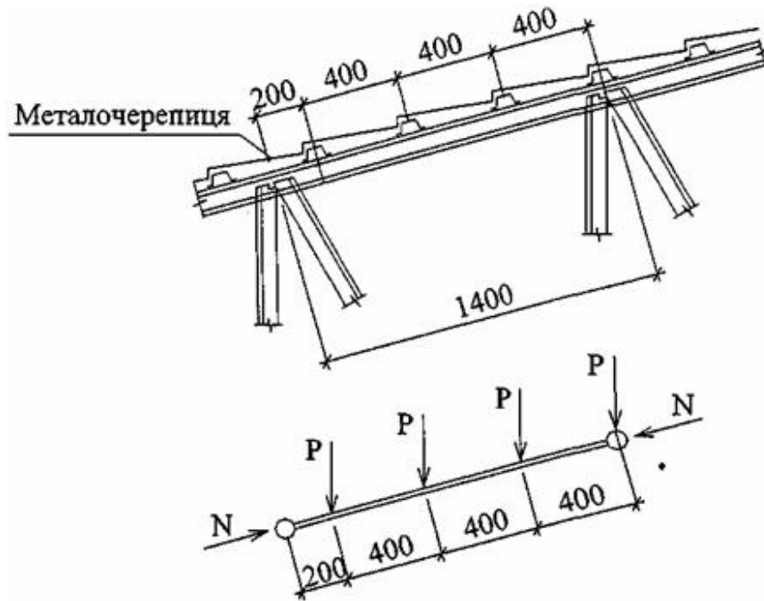
Рисунок В.2 – Навантаження верхнього поясу ферми
