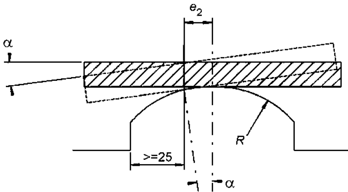
Рисунок 4 – Екцентриситет лінійного балансира Figure 4 – Line rocker eccentricity
