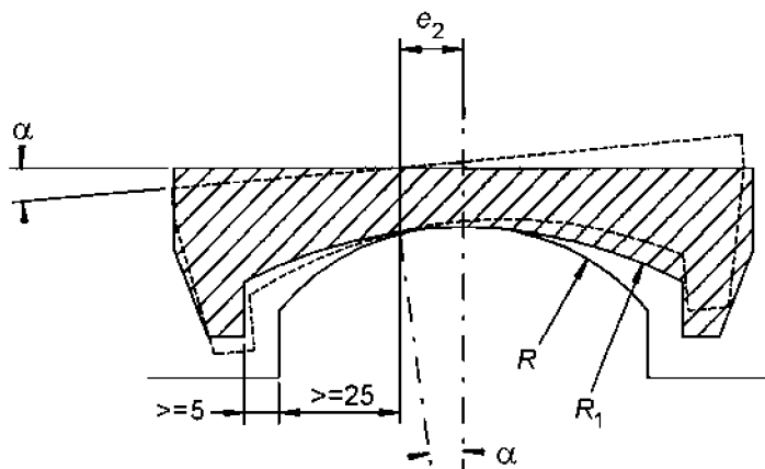
Рисунок 5 – Екцентриситет точкового балансира Figure 5 – Point rocker eccentricity
