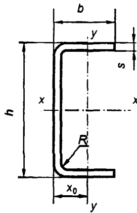
Рисунок 1 — Поперечний переріз швелера
