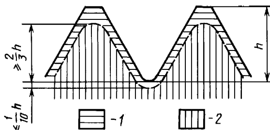
1 — полностью или частично обезуглероженная зона; 2 — необезуглероженная зона
