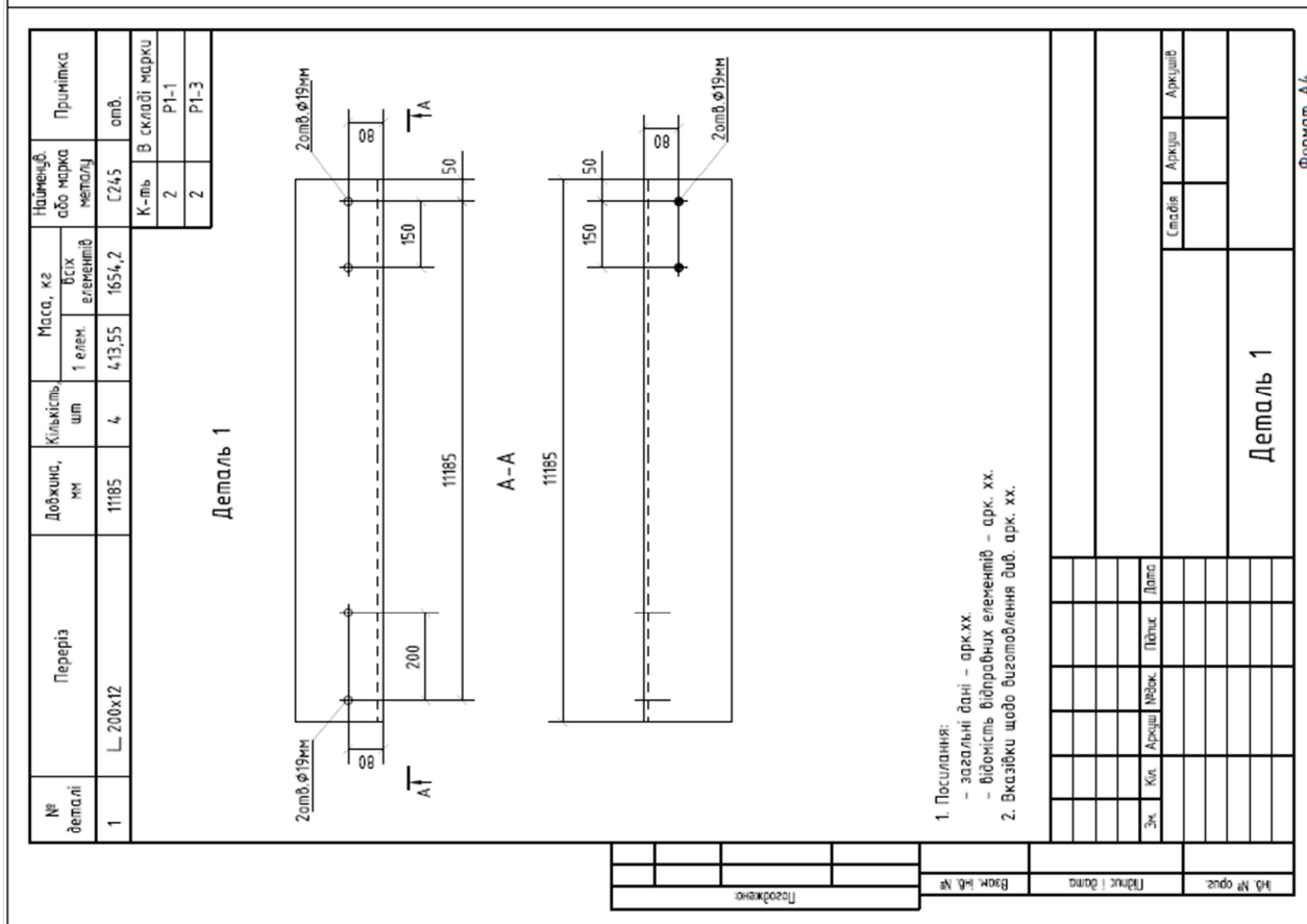
Рисунок Д.11, Д12 – Приклади оформлення деталей (прокатні профілі)
