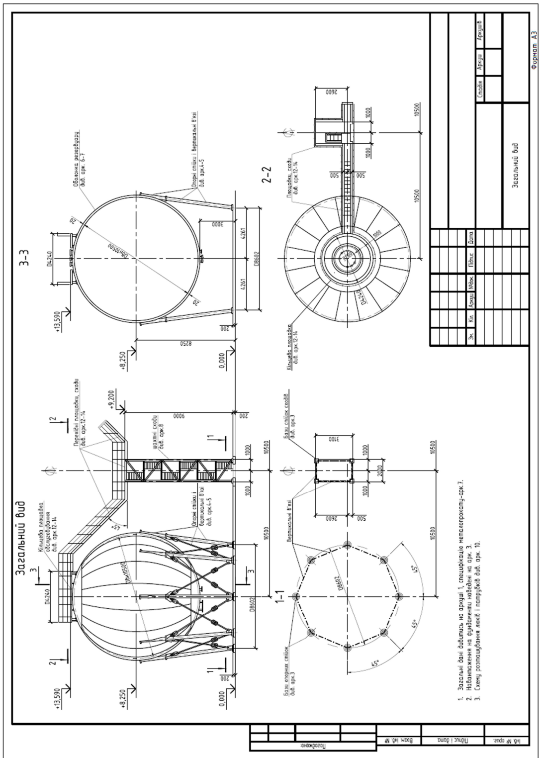
Рисунок Д.1 – Приклад оформлення аркуша загального виду
