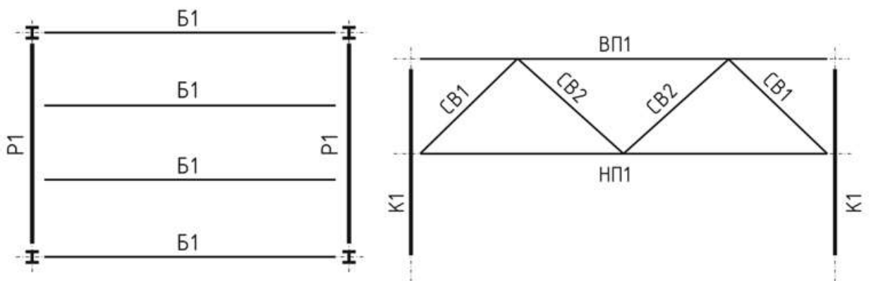
Рисунок 9.1. Схематичне зображення
