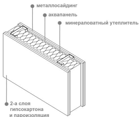
Конструкція зовнішніх стінових панелей
